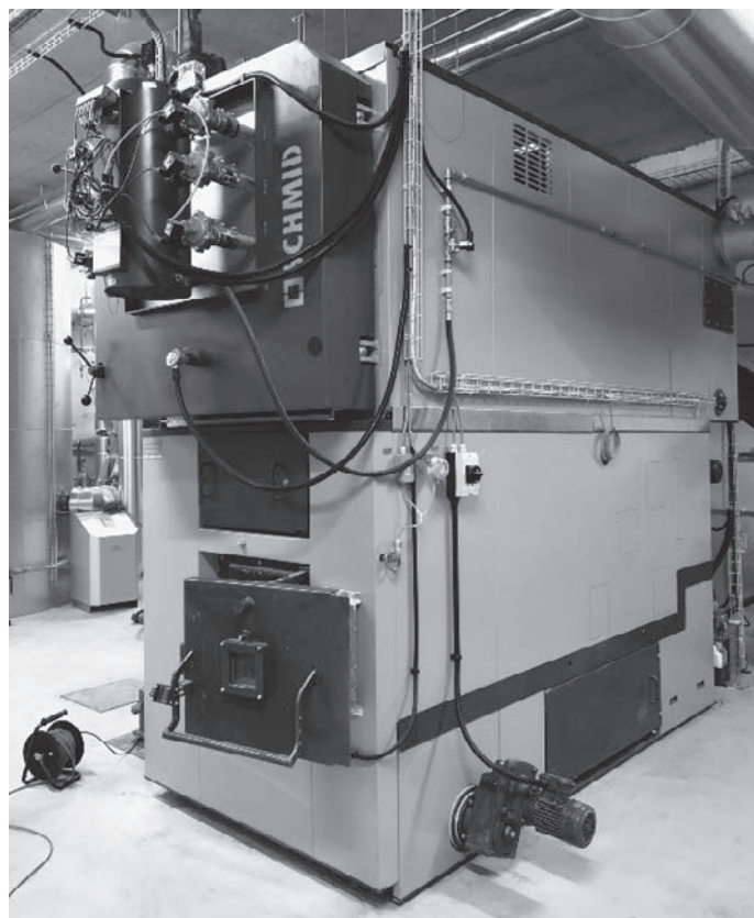
Holz hackschnitzelofen 550 kW
